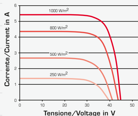
Esempio per/Example for AC-183M/125-72S
